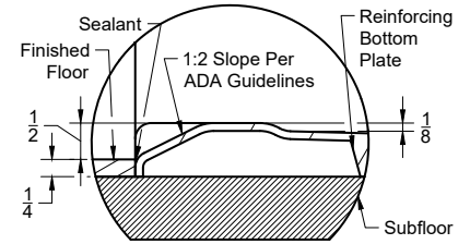
No-Recess
