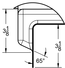
Return Flange
